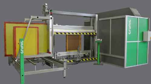
G-COAT 415 IN-LINE, liniowy system do nanoszenia emulsji, z szafą suszącą
